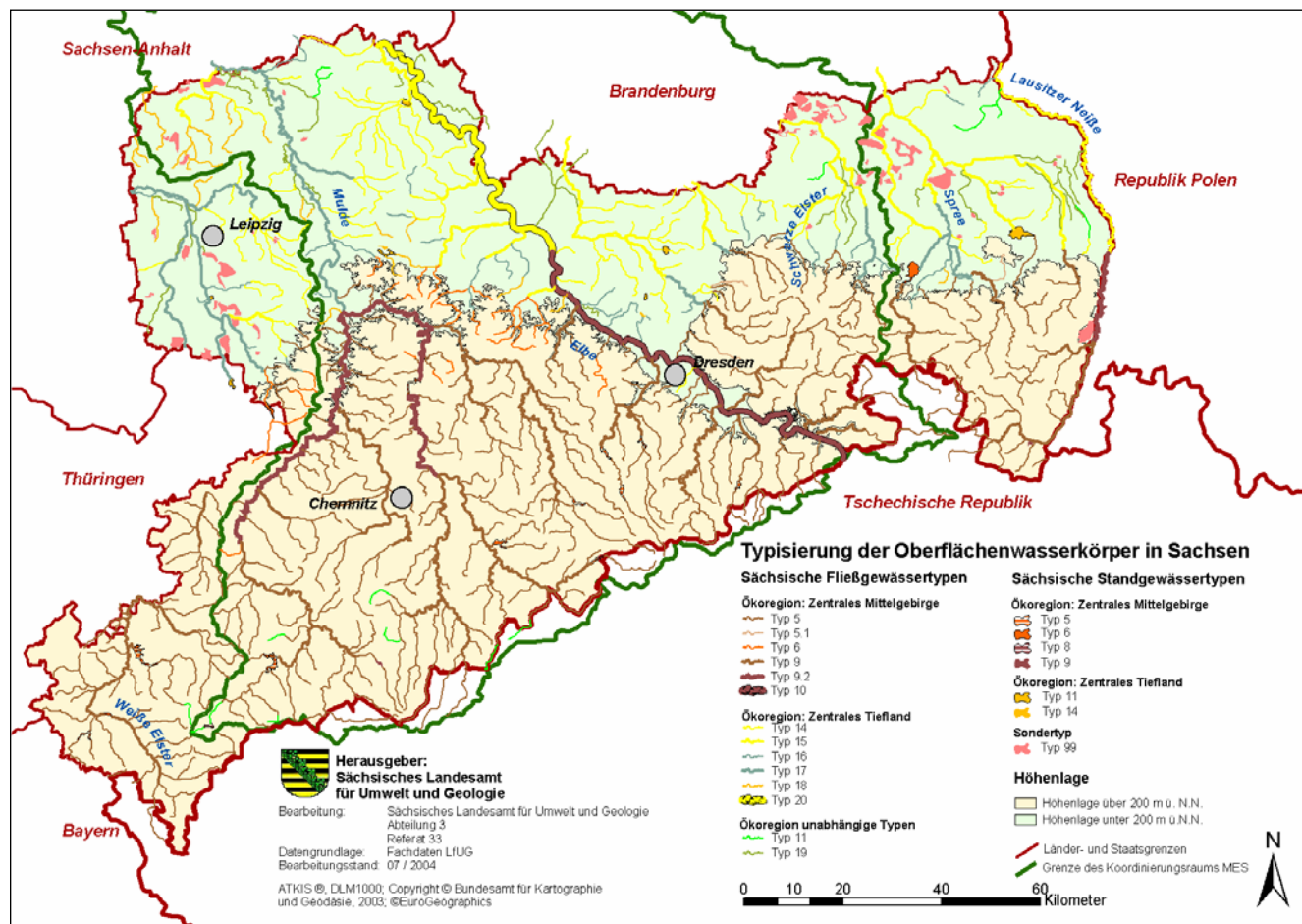
Übersicht zur Typisierung der Oberflächenwasserkörper in Sachsen
