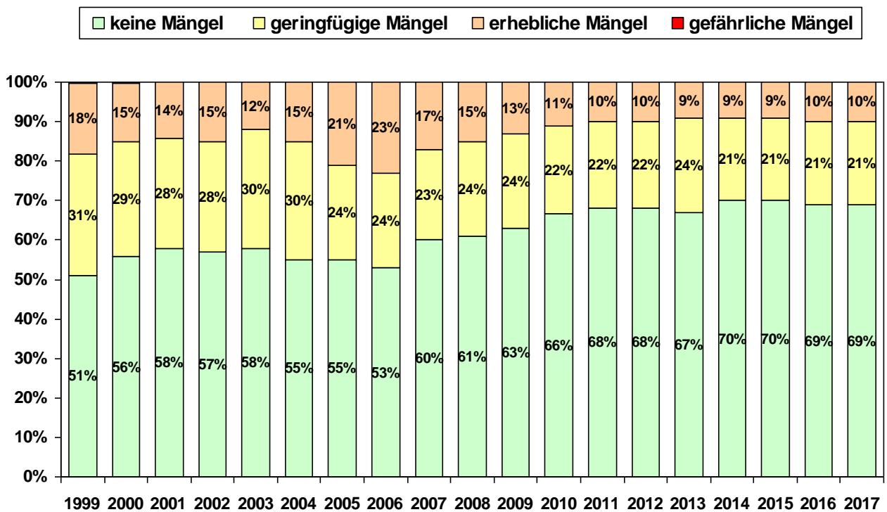
Abbildung 4: Verteilung der Mängelarten bei Prüfungen insgesamt
