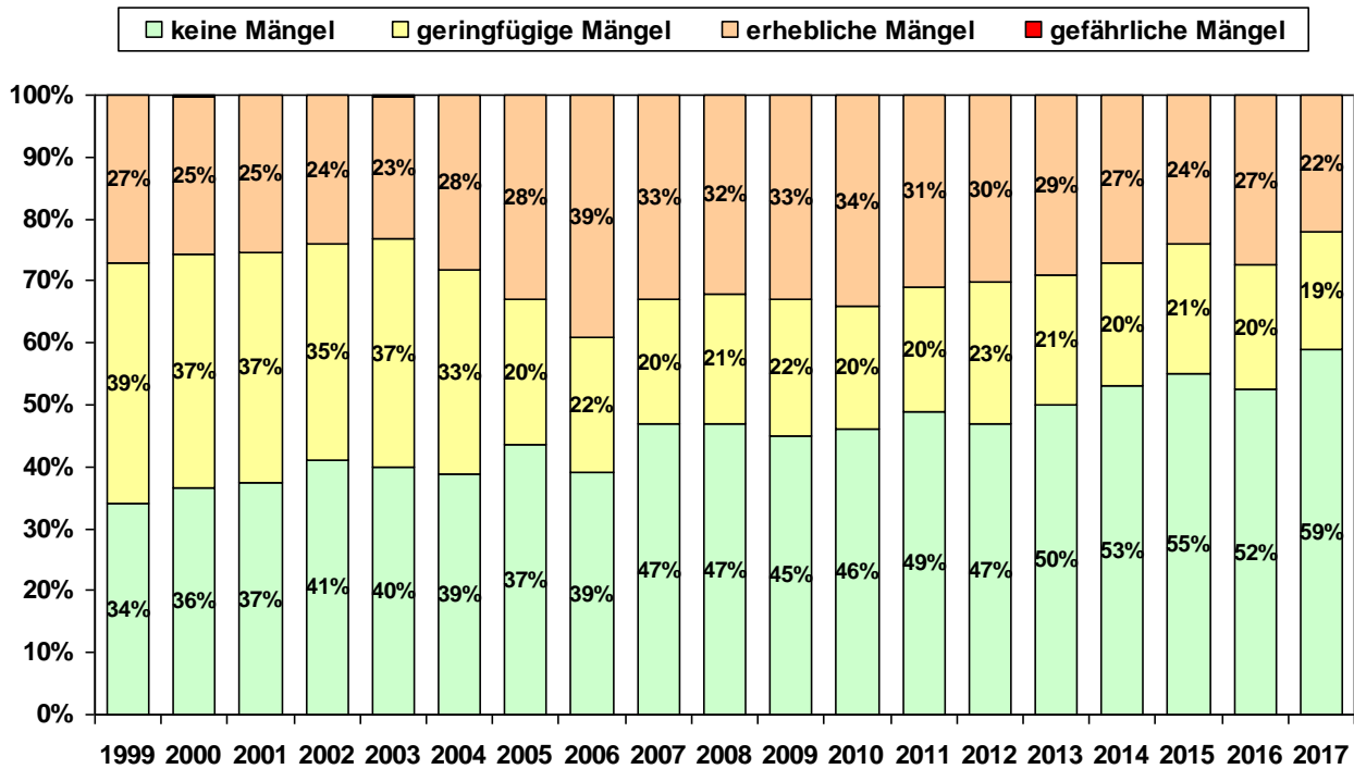
Abbildung 7: Mängelverteilung bei Heizölverbraucheranlagen (HVA) - Erstprüfungen
