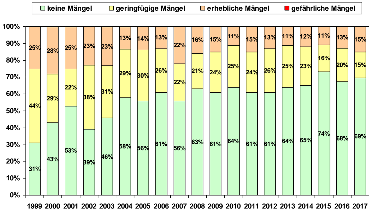
Abbildung 9: Mängelverteilung bei HBV-Anlagen - Erstprüfungen
