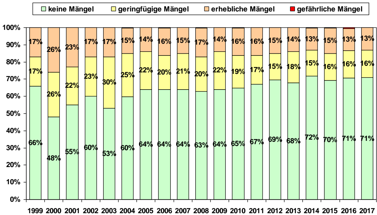
Abbildung 11: Mängelverteilung bei Tankstellen (TS) - Erstprüfungen
