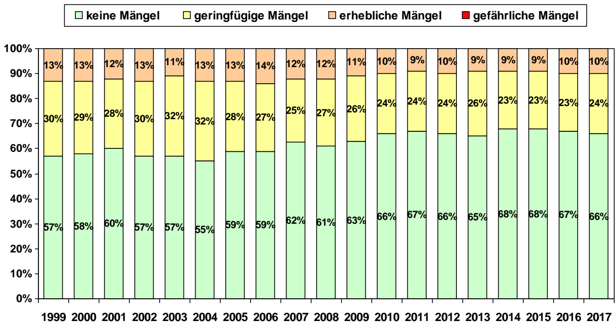
Abbildung 6: Verteilung der Mängel bei wiederkehrenden Prüfungen
