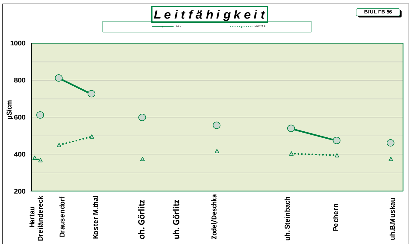
Abbildung 2: : Leitfähigkeit in \mu\text{S}/\text{cm} der Einzelmessungen August 2026 (links) und dem Jahresmittelwert 2025 (MW 25 li)
