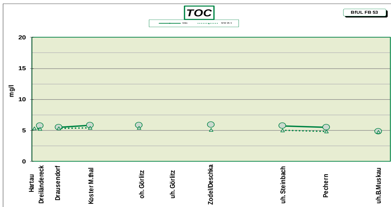
Abb. 4: TOC in mg/l der Einzelmessungen August 2026 (links) und dem Jahresmittelwert 2025 (MW 25 li)
