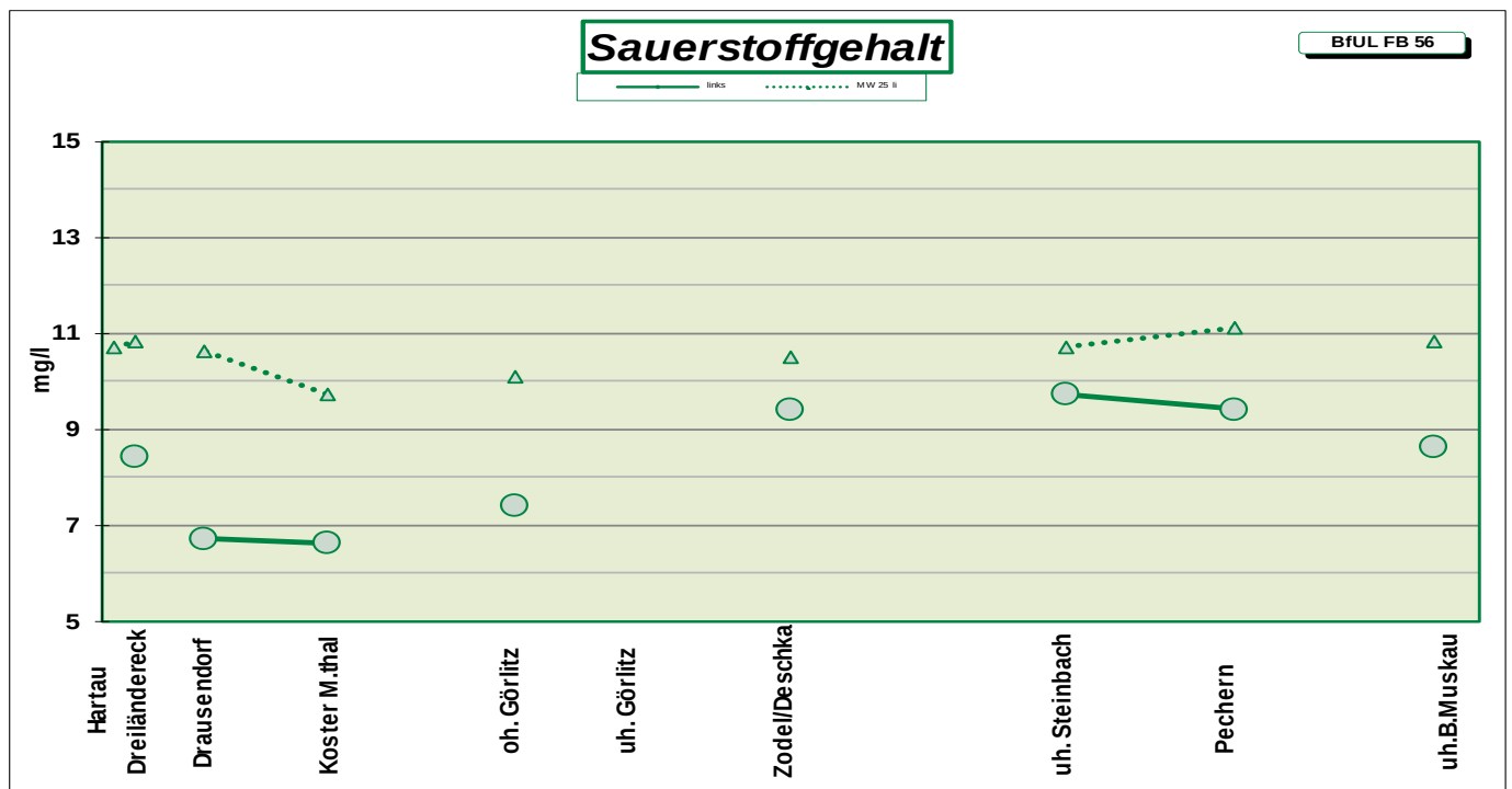
Abbildung 1: Sauerstoffgehalt in mg/l der Einzelmessungen August 2026 (links) und dem Jahresmittelwert 2025 (MW 25 li)
