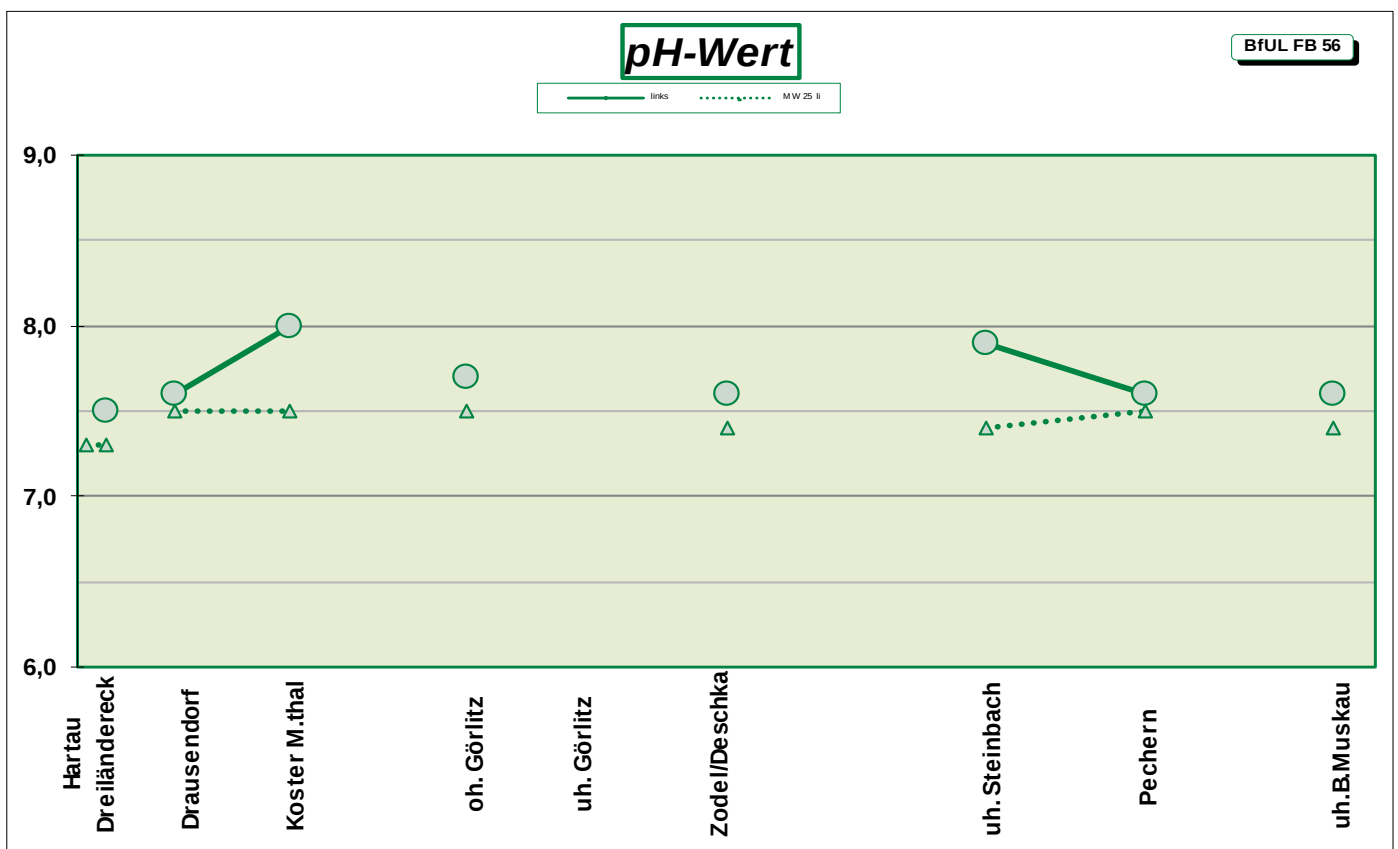
Abb. 3: pH-Werte aus den Einzelmessungen August 2026 (links) und dem Jahresmittelwert 2025 (MW 25 li)
