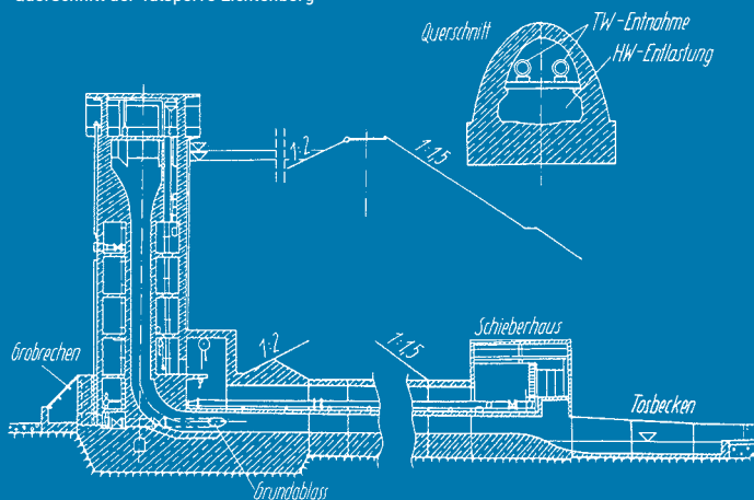
Querschnitt der Talsperre Lichtenberg
