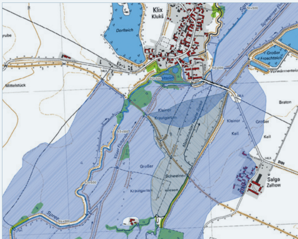
Abbildung 5-8: Ausbreitung der Überflutungsflächen zum Hochwasser im August 2010 südlich der Ortslage Klix (Quelle: Koban & Schuckert Ingenieurpartnerschaft 2012b)
