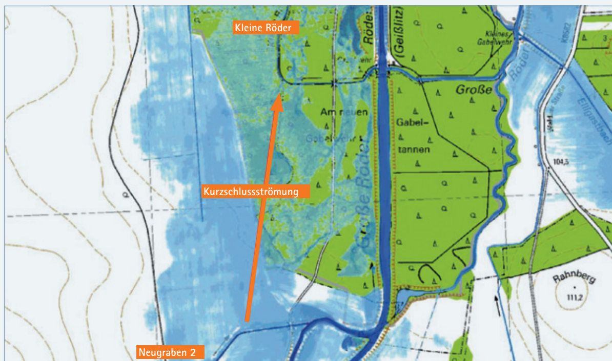
Abbildung 5-4: Die Kurzschlussströmung zwischen Neugraben 2 und Kleiner Röder beim Hochwasser im September 2010 (Quelle: Koban & Schuckert Ingenieurpartnerschaft 2012a)
