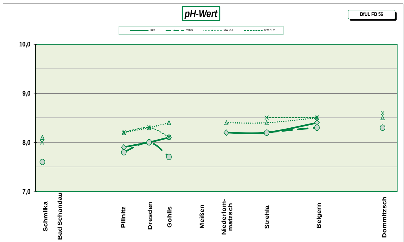
Abb. 3: pH-Werte aus den Einzelmessungen September 2026 (links, rechts) und dem Jahresmittelwert 2024 (MW 24 li, re)
