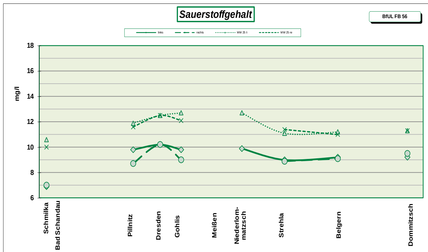
Abbildung 1: Sauerstoffgehalt in mg/l der Einzelmessungen September 2026 (links, rechts) und dem Jahresmittelwert 2025 (MW 25 li, re)
