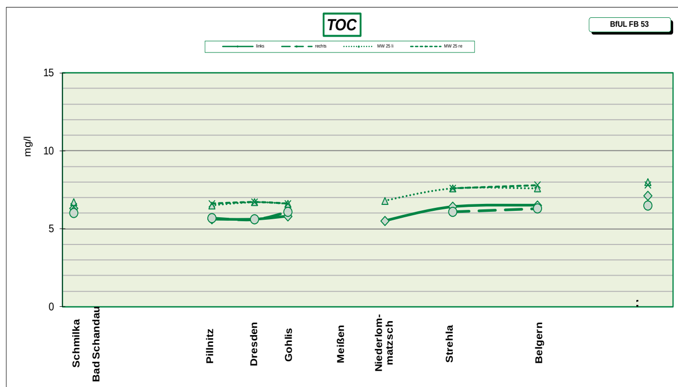
Abb. 4: TOC in mg/l der Einzelmessungen September 2026 (links, rechts) und dem Jahresmittelwert 2025 (MW 25 li, re)
