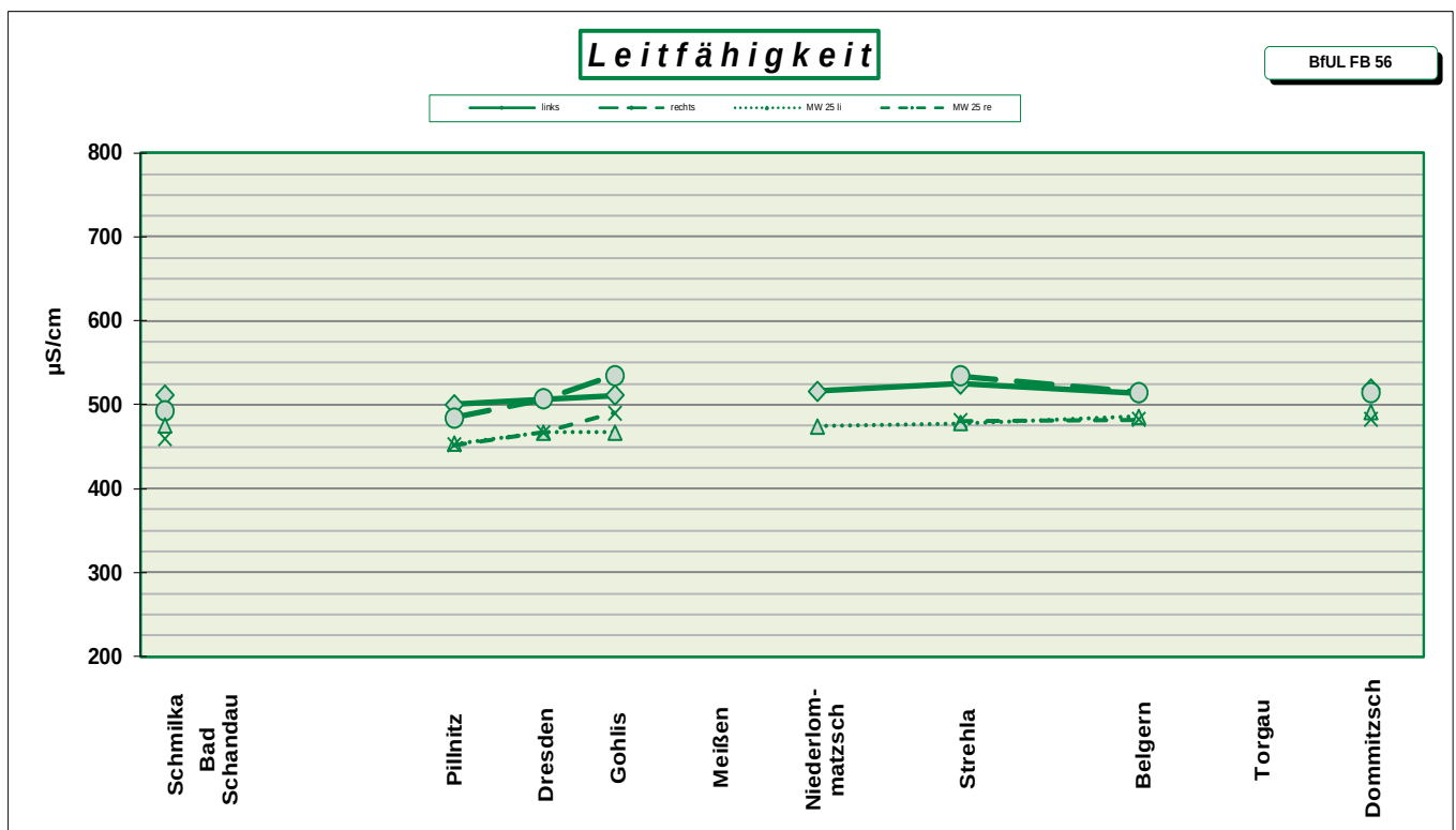
Abbildung 2: : Leitfähigkeit in \mu\text{S}/\text{cm} der Einzelmessungen September 2026 (links, rechts) und dem Jahresmittelwert 2025 (MW 25 li, re)
