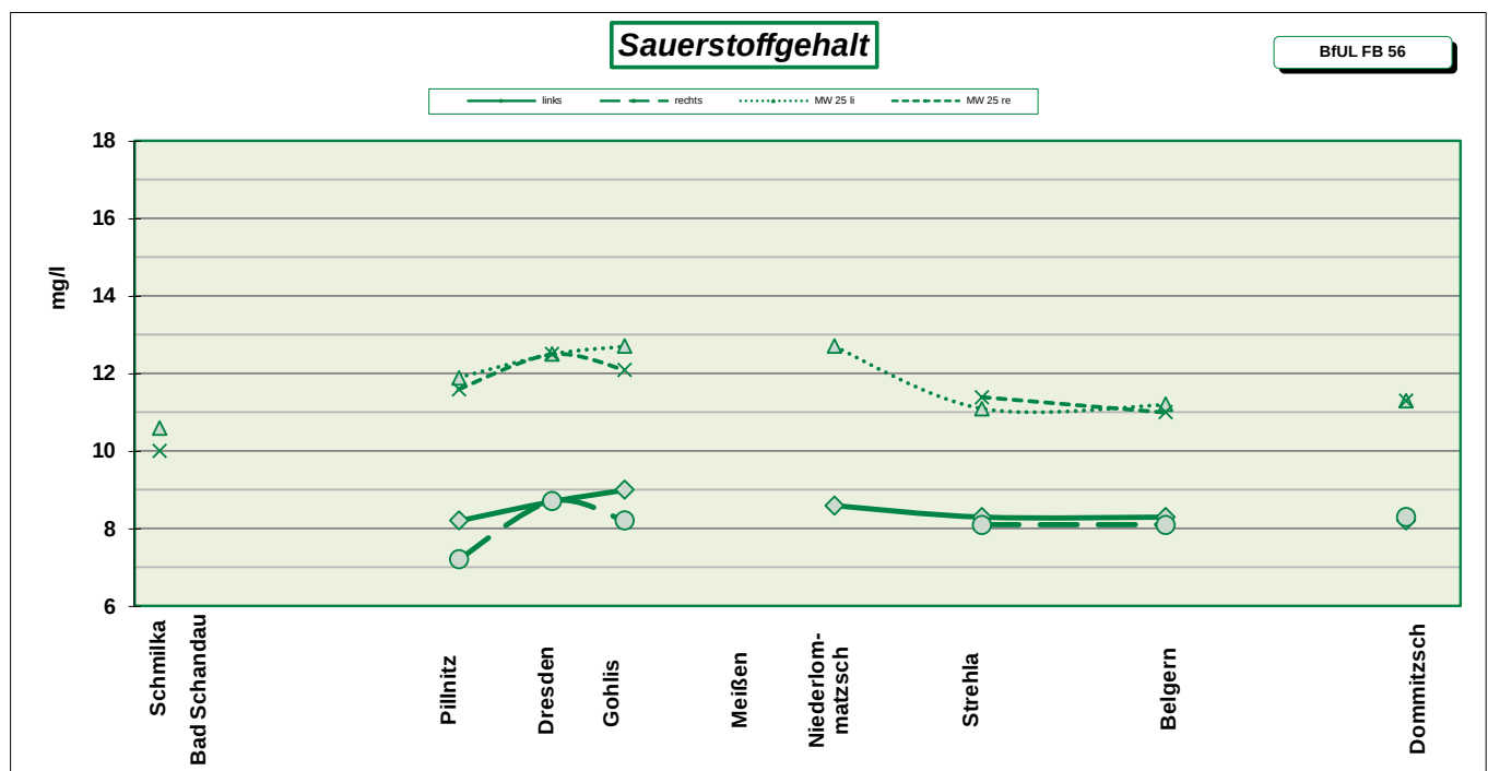
Abbildung 1: Sauerstoffgehalt in mg/l der Einzelmessungen Juli 2026 (links, rechts) und dem Jahresmittelwert 2025 (MW 25 li, re)
