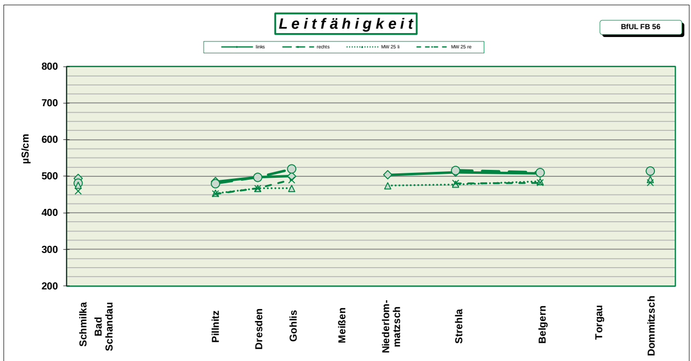
Abbildung 2: : Leitfähigkeit in \mu\text{S}/\text{cm} der Einzelmessungen Juli 2026 (links, rechts) und dem Jahresmittelwert 2025 (MW 25 li, re)
