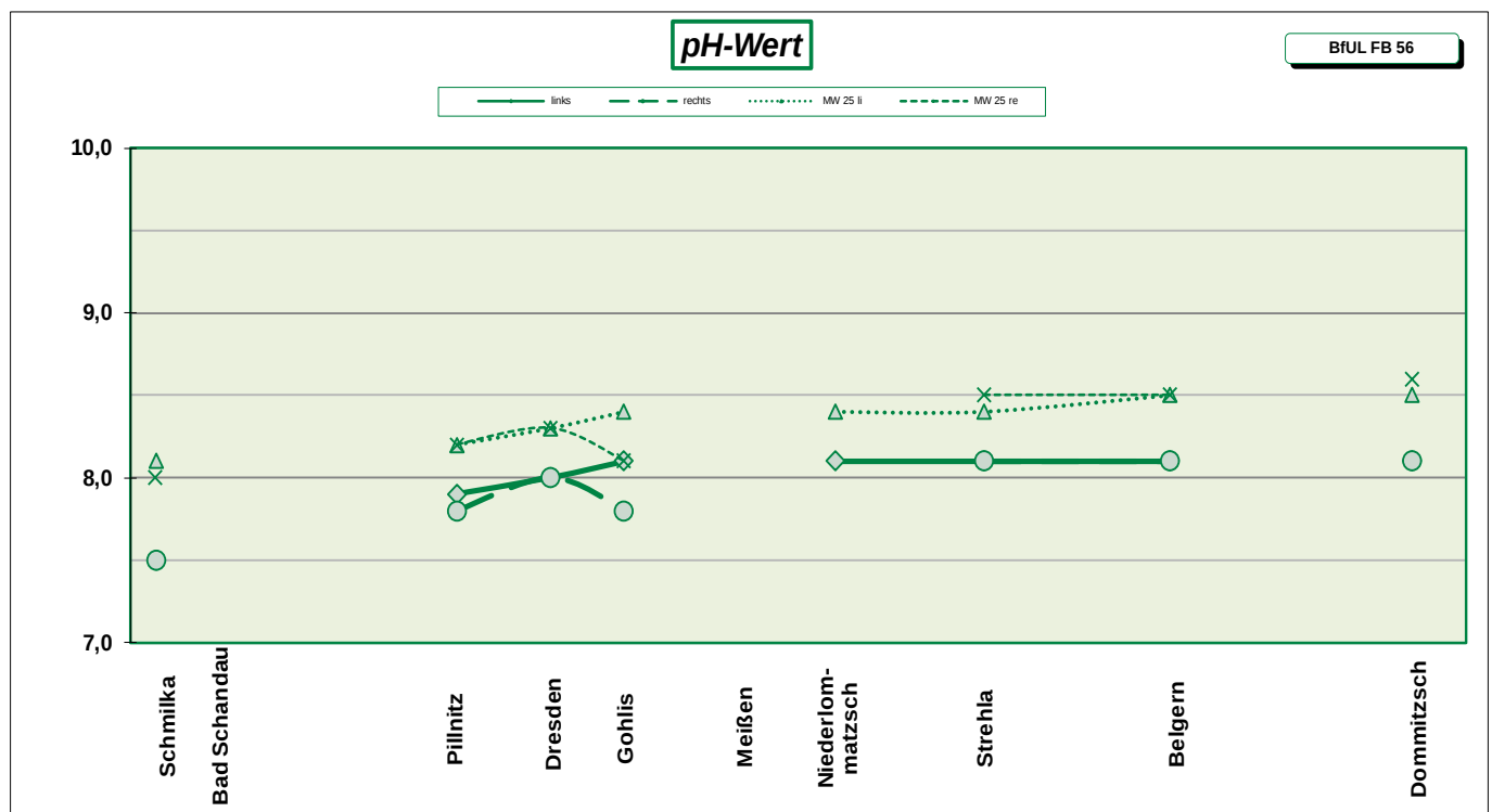
Abb. 3: pH-Werte aus den Einzelmessungen Juli 2026 (links, rechts) und dem Jahresmittelwert 2024 (MW 24 li, re)
