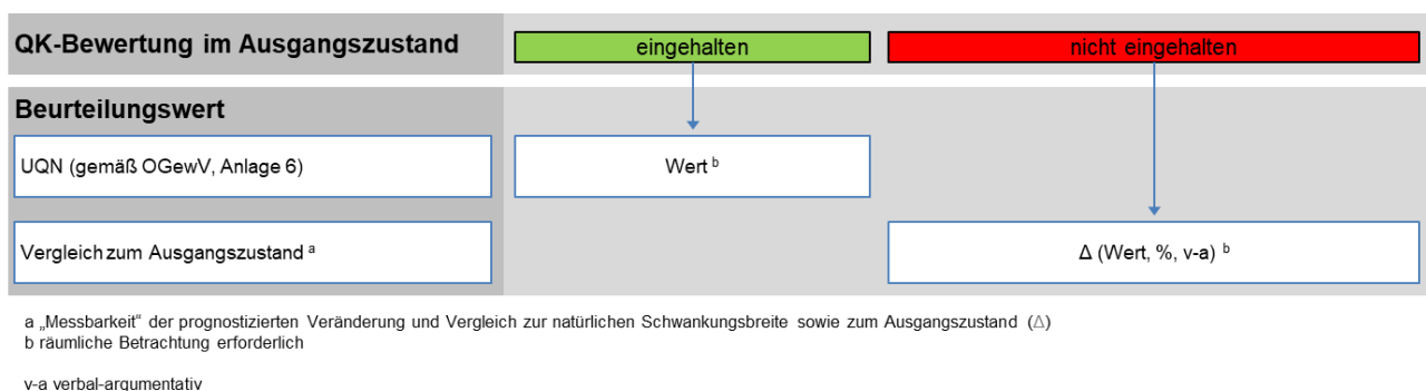
Abbildung 2: Fließschema zur Ermittlung der relevanten Prüfansätze für flussgebiets-spezifische Schadstoffe in Abhängigkeit vom Ausgangszustand der jeweiligen UQN
