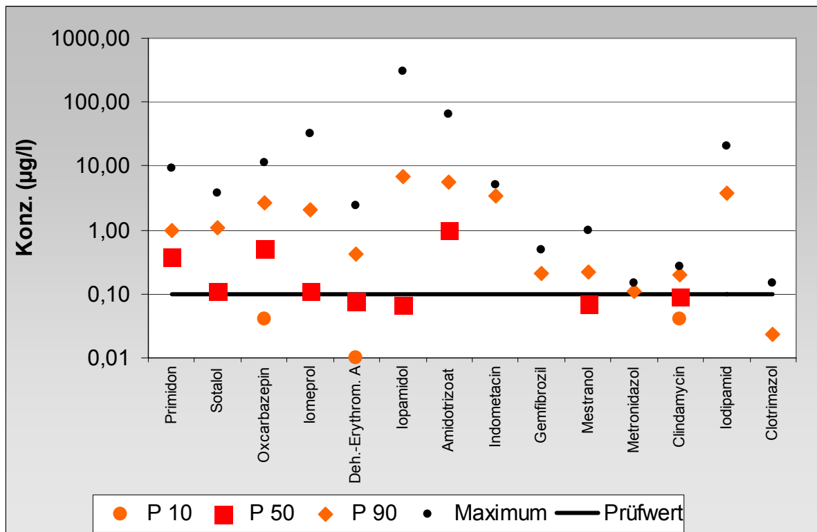
Abbildung 2: 10-Perzentil, Median (P50), 90-Perzentil (P90) und Maximum (Max) aus allen Kläranlagenuntersuchungen für Arzneistoffe, die im Ablauf kommunaler Kläranlagen in Konzentrationen über dem Prüfwert (0,1 µg/L) gemessen wurden
