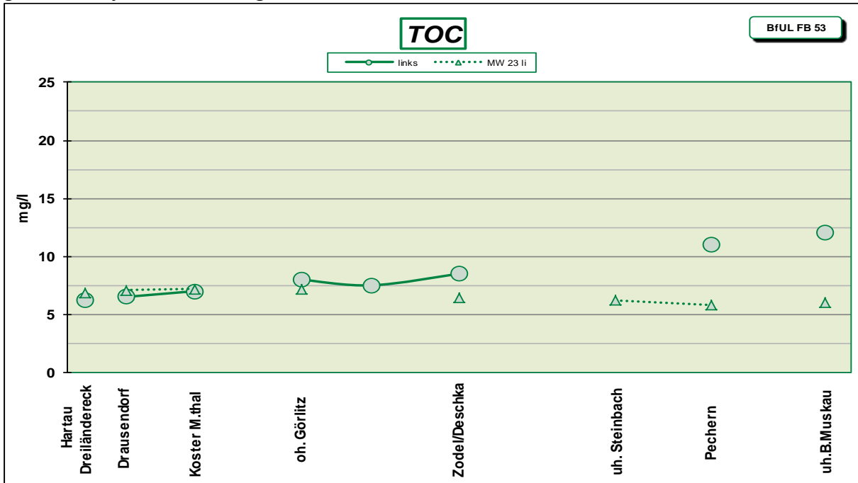
Abb. 4: Mittelwerte des TOC in mg/l aus den Messungen Februar 2024 (links) und Februar 2023 (MW 22 li)
