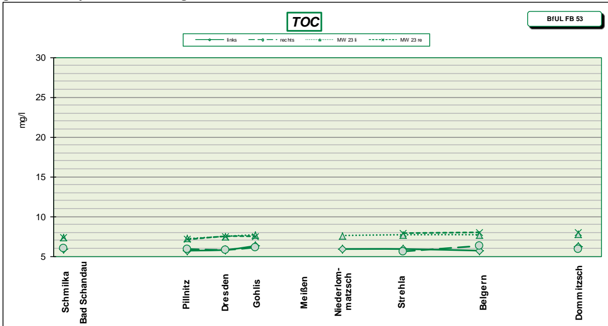
Abb. 4: Mittelwerte des TOC in mg/l aus den Messungen März 2024 (links, rechts) und März 2023 (MW 23 li, re)
