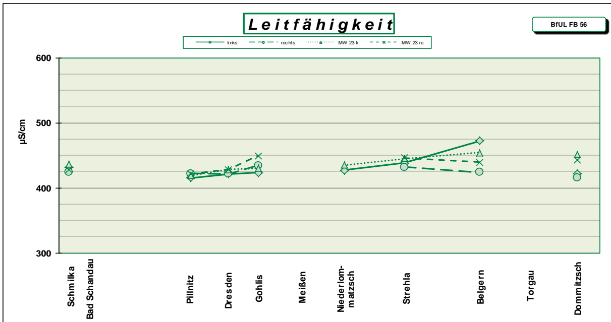
Abb. 2: Mittelwerte der Leitfähigkeit in \mu\text{S}/\text{cm} aus den Messungen März 2024 (links, rechts) und März 2023 (MW 23 li, re)
