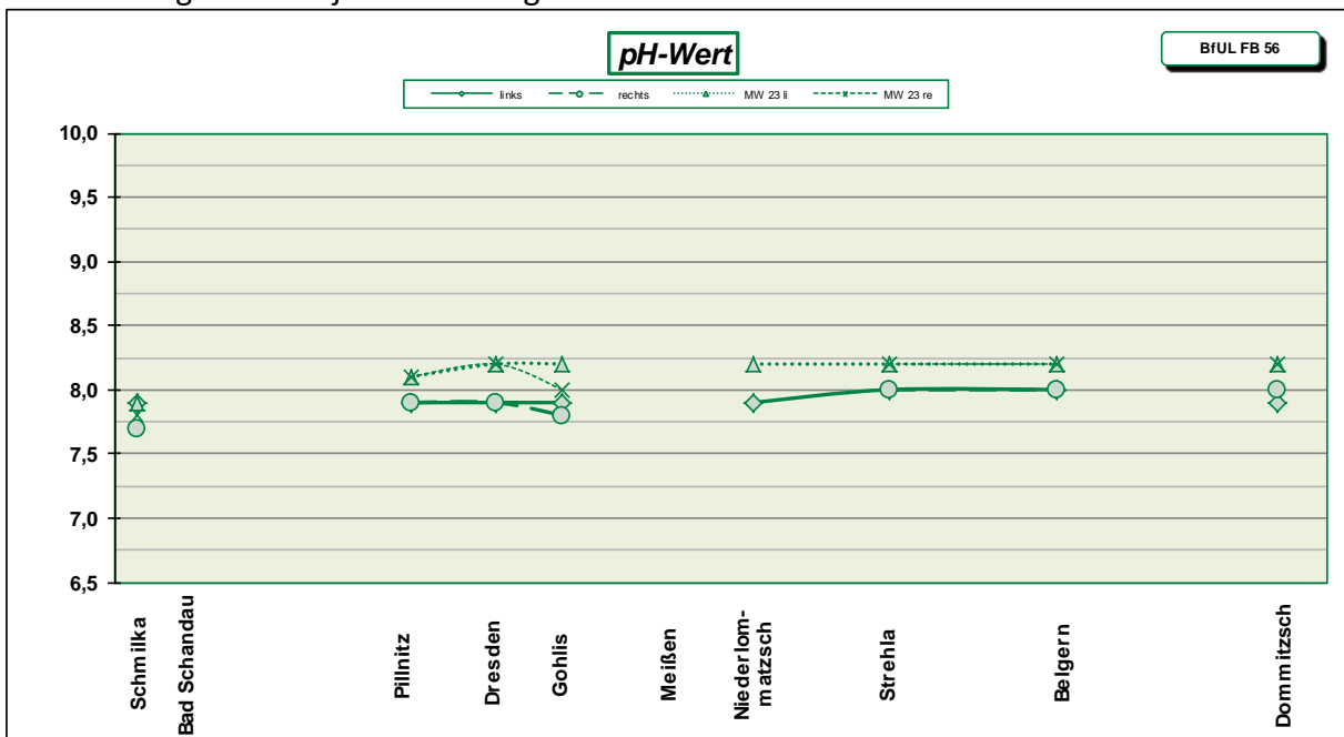
Abb. 3: Mittelwerte der pH-Werte aus den Messungen März 2024 (links, rechts) und März 2023 (MW 23 li, re)
