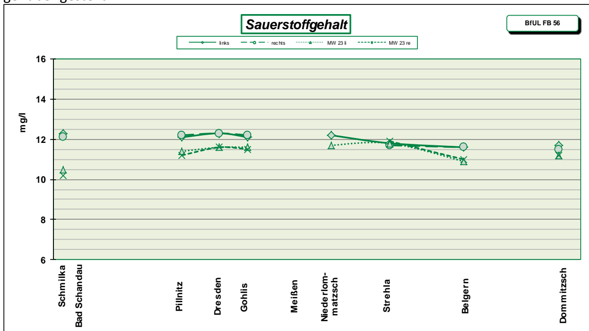
Abb. 1: Mittelwerte des Sauerstoffgehalts in mg/l aus den Messungen März 2024 (links, rechts) und März 2023 (MW 23 li, re)
